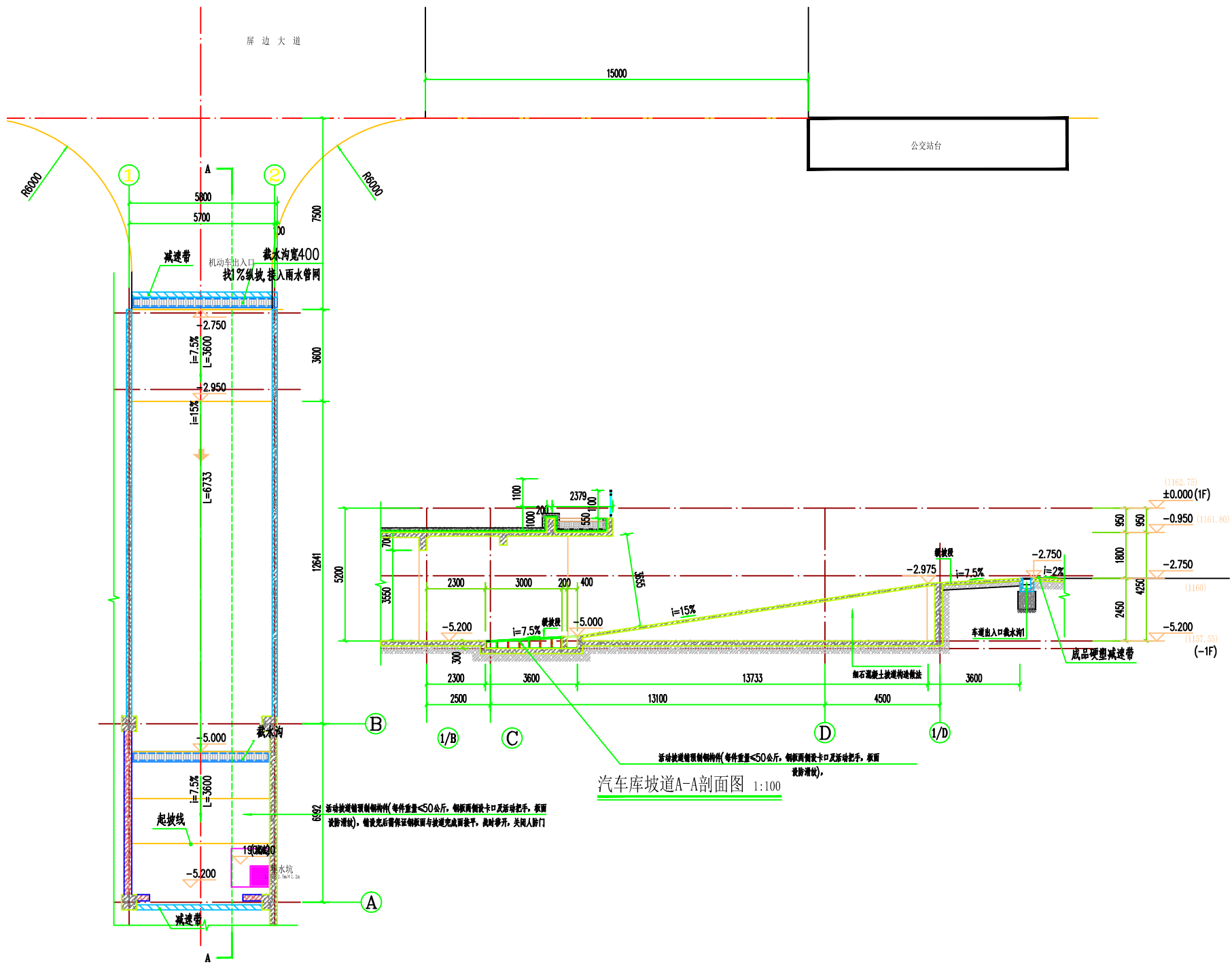
汽车库坡道首层平面图 1:100
